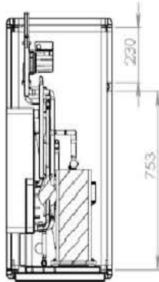
A-A (1 : 15)
